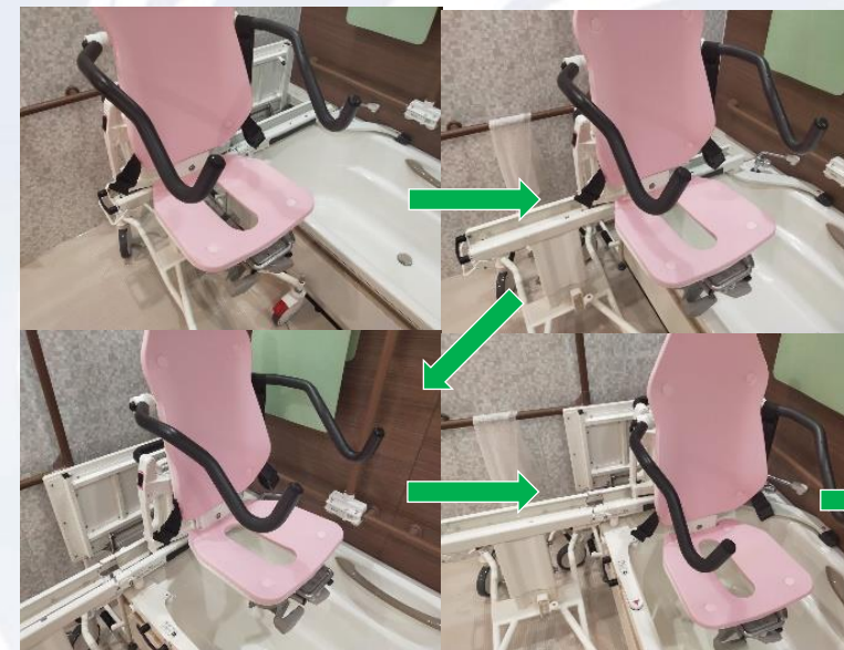
入浴用車椅子
